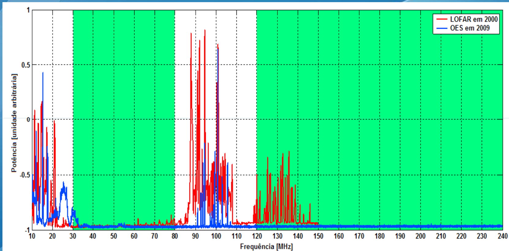
Figura 1. – Característica do Espectro Eletromagnético em observações no OES/CRS/CCR/INPE-MCT, em 2009 (10 – 240 MHz), em comparação com os dados Espectrais medidos em uma estação do LOFAR (10 – 150 MHz), publicado por Boonstra et al. (2000). A magnitude dos sinais não está na escala. O intervalo de operação do LOFAR está em verde. Fonte: Rosa (2009).
