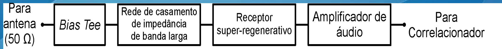
Figura 5 – Topologia básica do receptor proposto.
