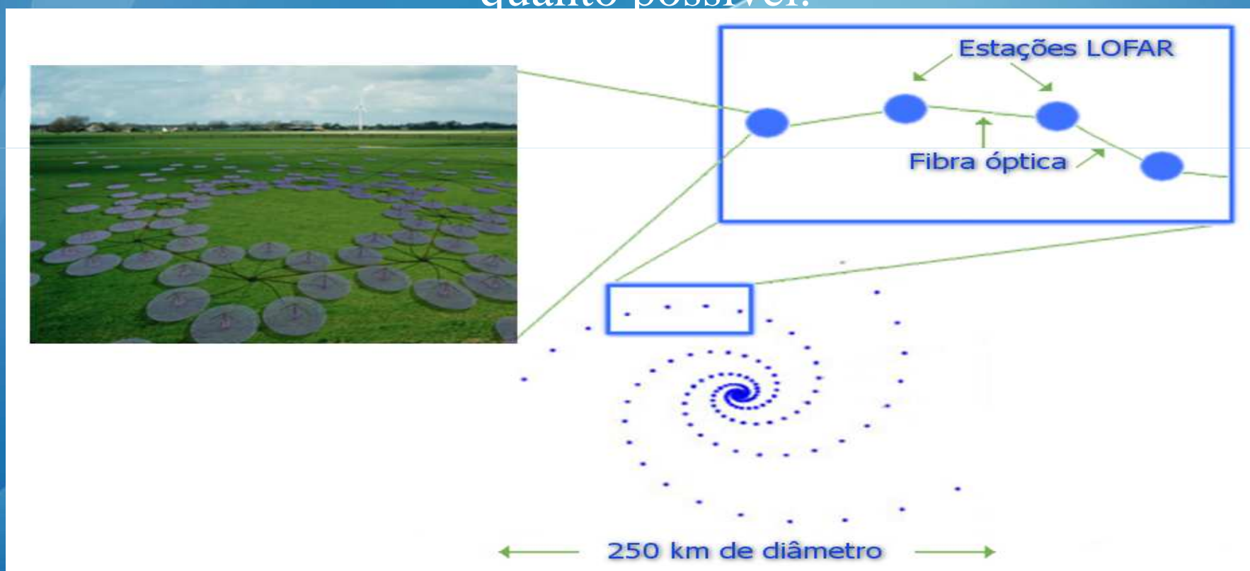
Figura 3. Subsistema do LOFAR.
