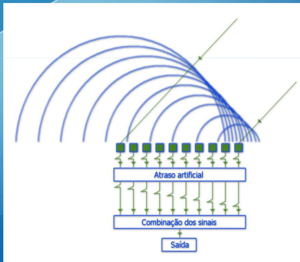
Figura 2 e 2.1 – Comparação entre um radiotelescópio convencional e sistema de defasagem utilizado no LOFAR
